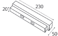
Блок питания 200W / 48V Цвет — черный
