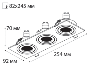
SAG 303-4
