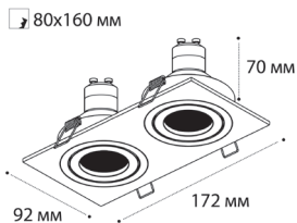
SAG 203-4
