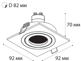
SAG 103-4
